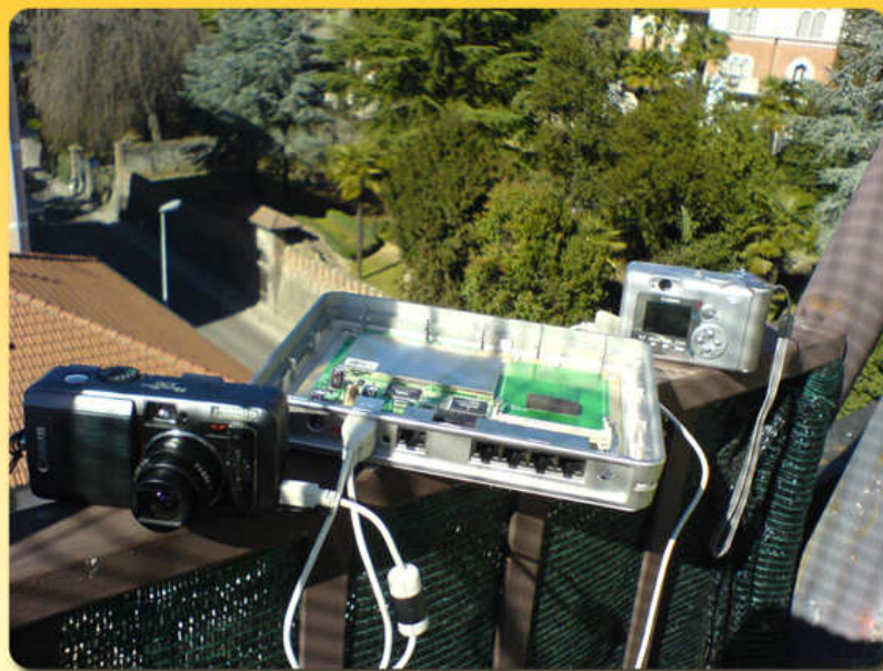
Asus WL-500gP Firmware OpenWRT Software gphoto2 per applicazione webcam
